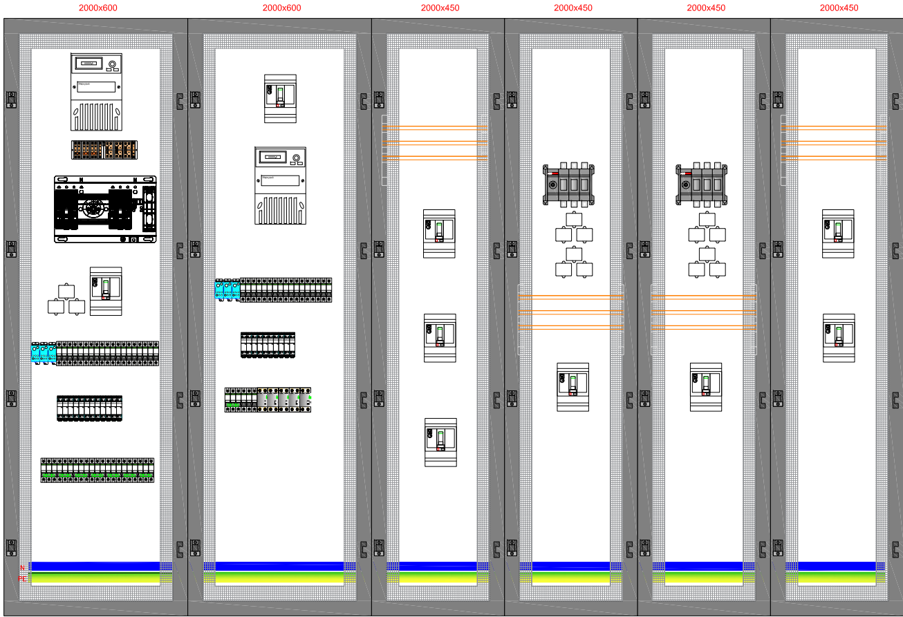
Щит ВРУ1 ВхШхГ=2000х3000х450мм
