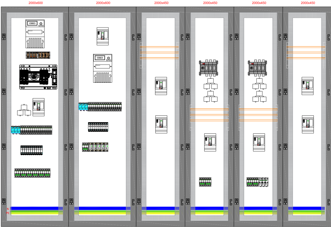
Щит ВРУ2 ВхШхГ=2000х3000х450мм
